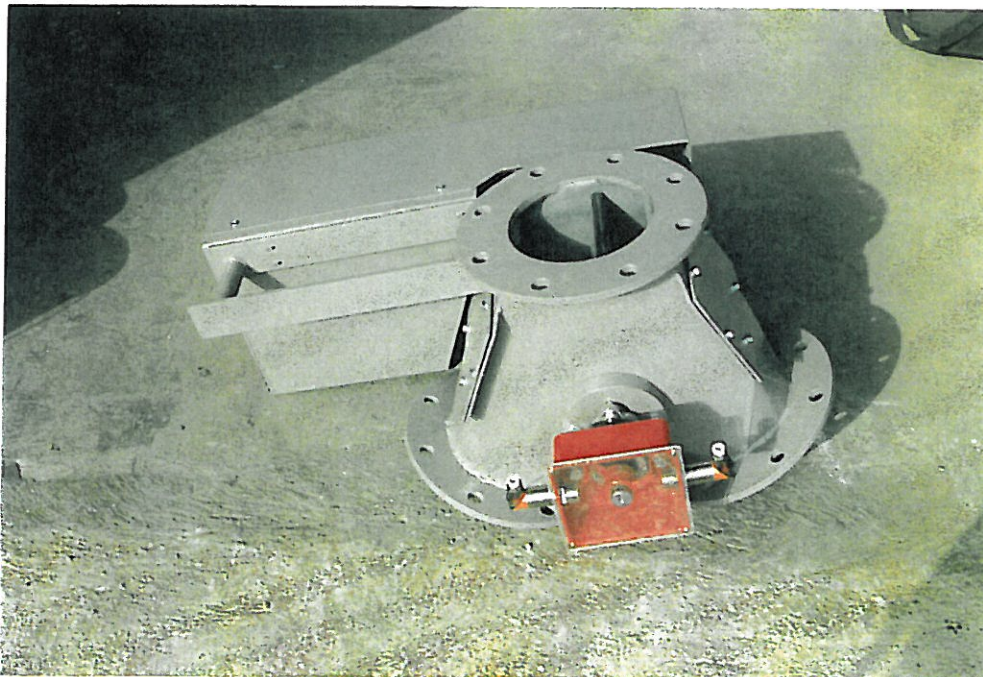
Zweiwegeverteiler rund symmetrisch mit Handhebel
