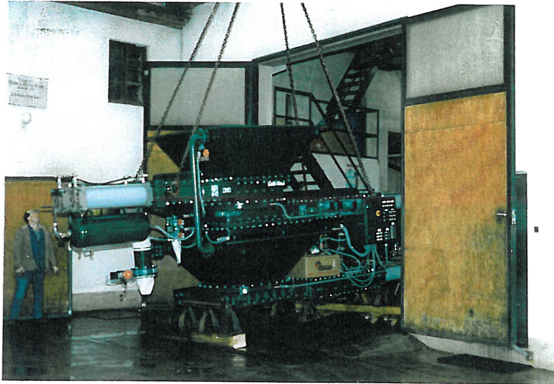
Taktchleuse DN 1000 für Differenzdruck 2,5 bar, Taktzeit 25 sek., Antrieb über 2 Stück Druckluftzylindern D=250 mit zusätzlichem Materialabsperrschieber
